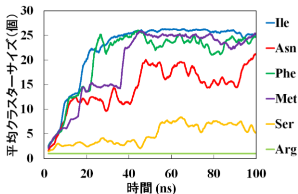
図 1 各アミノ酸の平均クラスターサイズ
