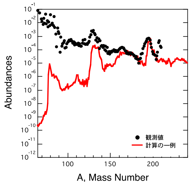
図 1 7900 種類の核種を用いた核反応ネットワーク計算の一例。
