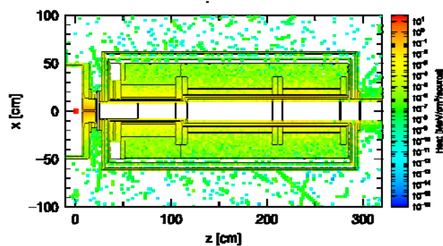
図 1 生成標的直後の超伝導電磁石における熱負荷分布
